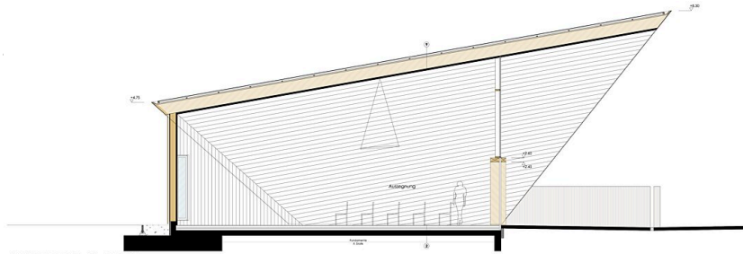
SCHNITT E-E, M. 1:100 (Gebüdeteile in die Bildebene gedreht)
