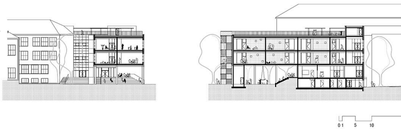
Schnitte
