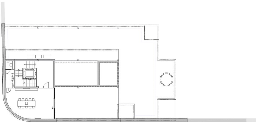
Grundriss DG
