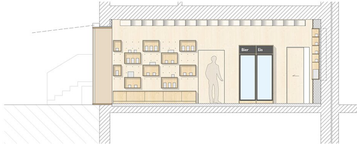
SCHNITT D - D M 1:50
