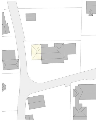
LAGEPLAN M 1:500
