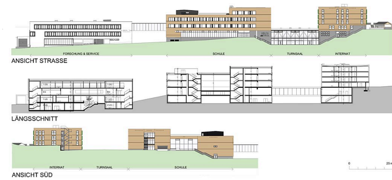
Ansichten Schnitte
