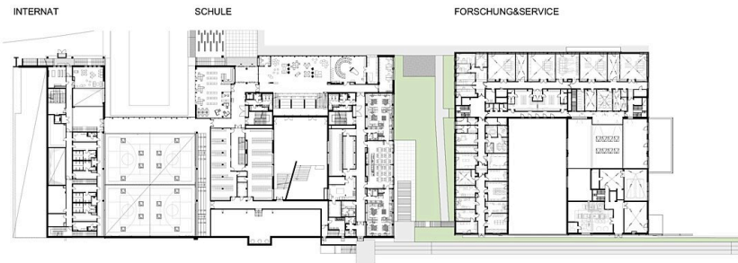
ERDGESCHOSS
