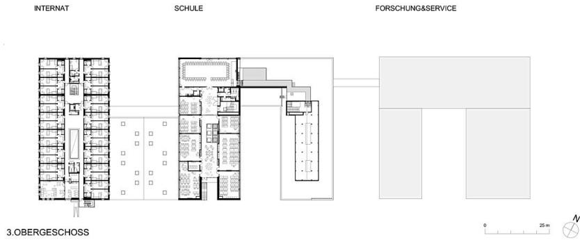
Grundriss OG3
