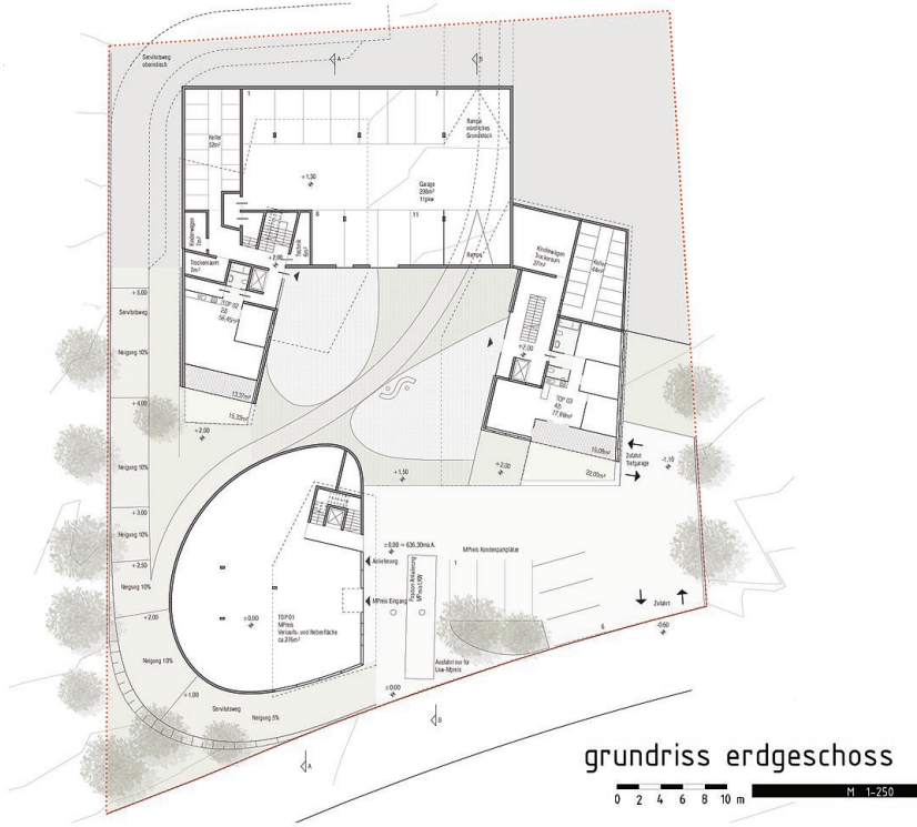
Grundriss EG
