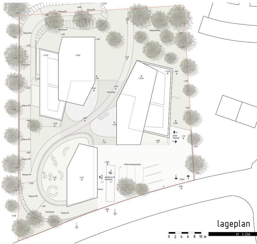
Lageplan
