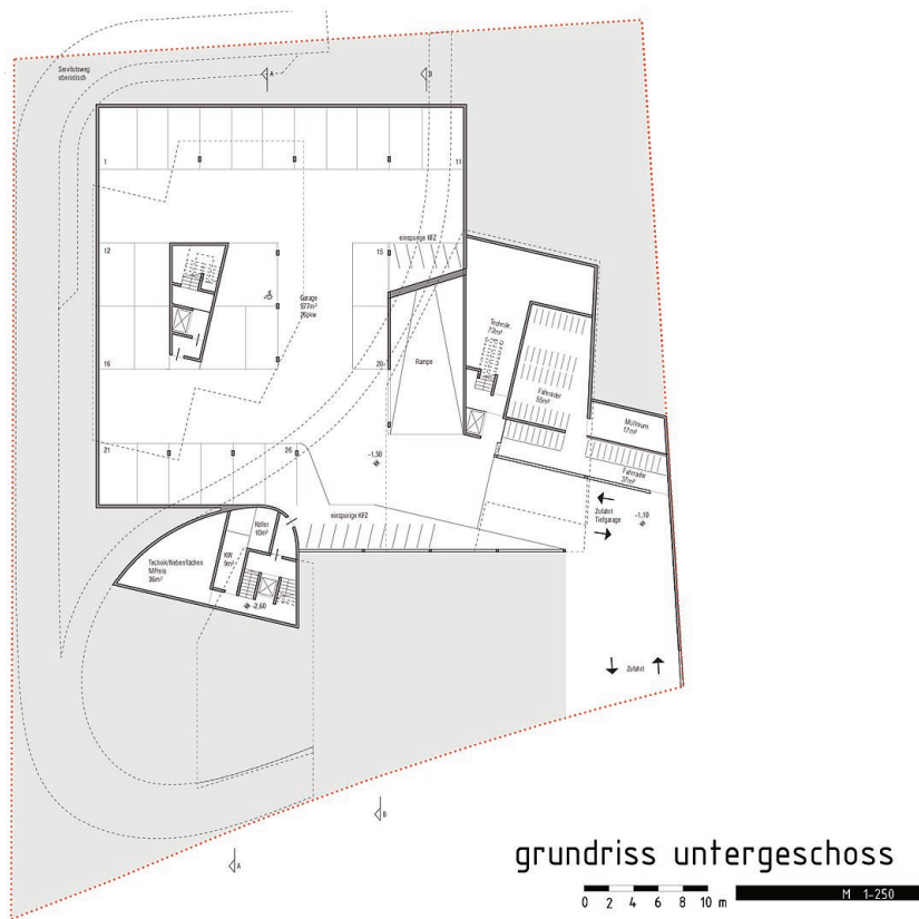
Grundriss UG
