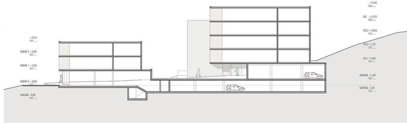
SCHNITT AA
