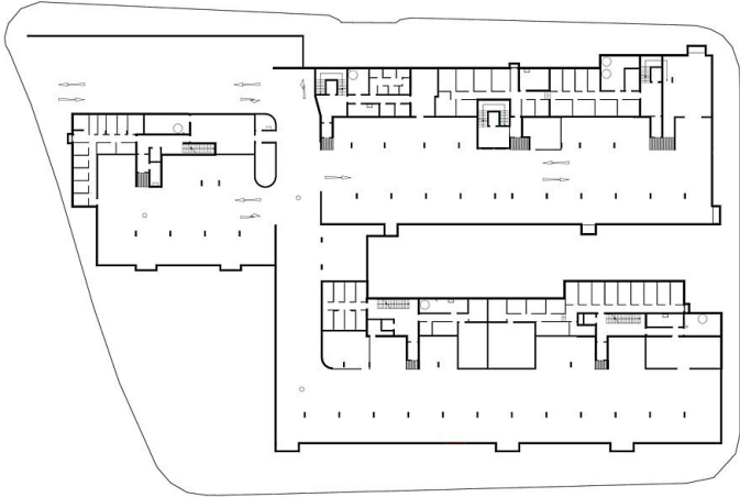
Untergeschoss 1:500
