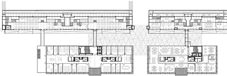
Grundriss OG3
