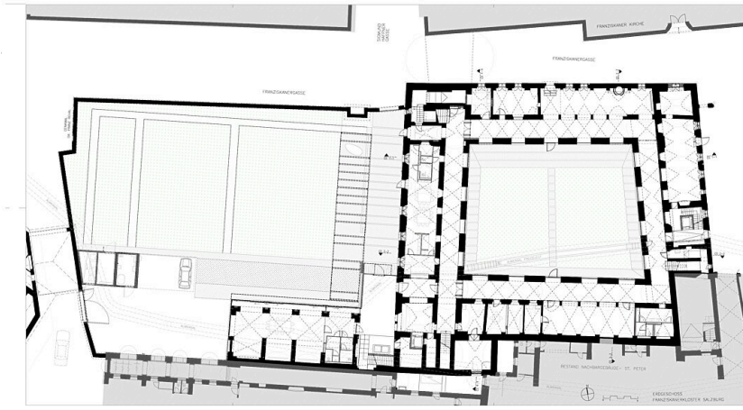
Grundriss EG
