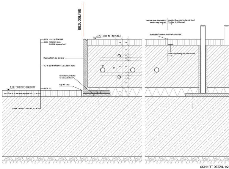
SCHNITT DETAIL 1:2
