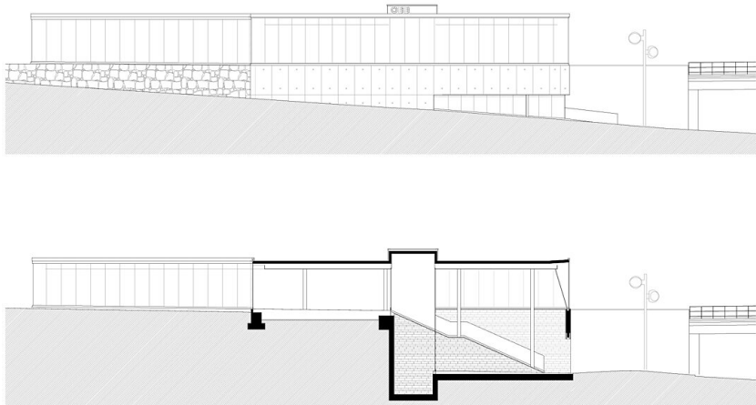
Schnitt, Ansicht
