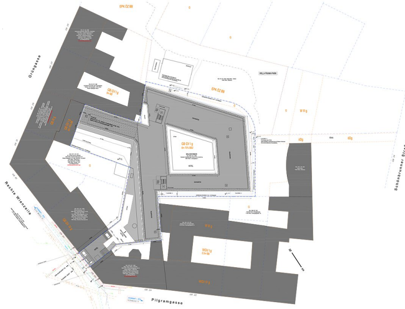
lageplan 1:250
