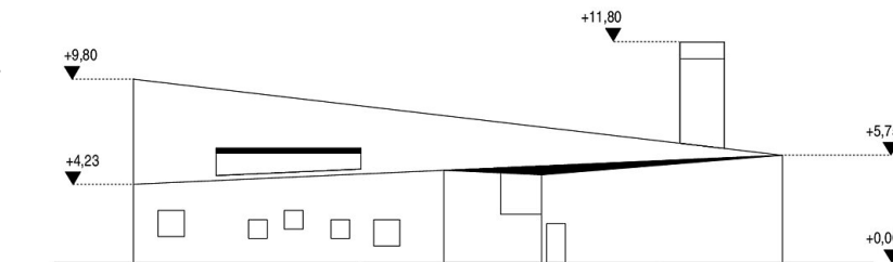
Ansicht Nordost
