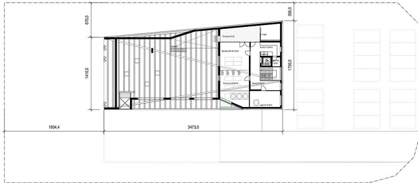
Grundriss Obergeschoss
