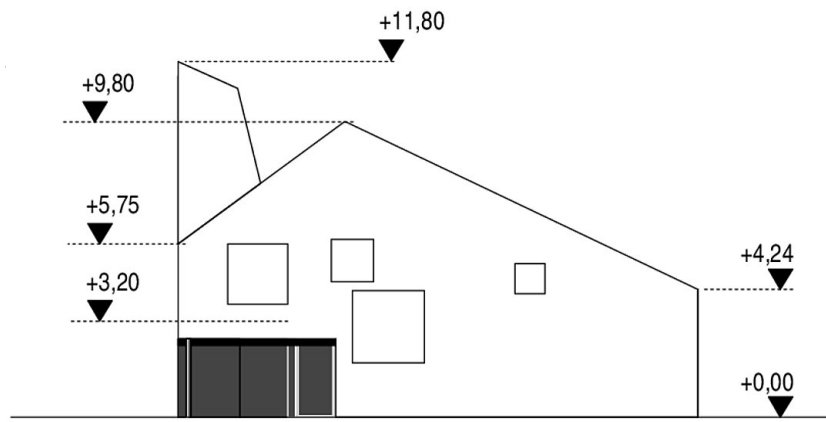
Ansicht Südost
