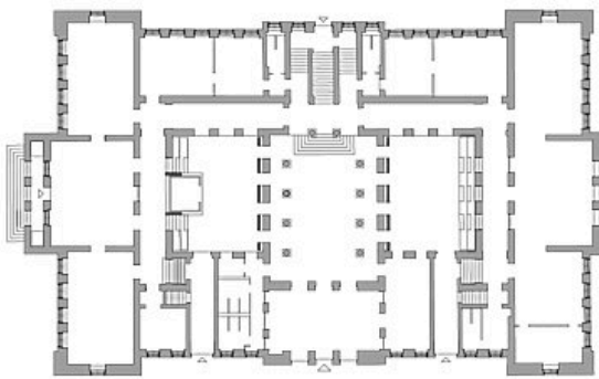
GRUNDRISS EG M 1:200
