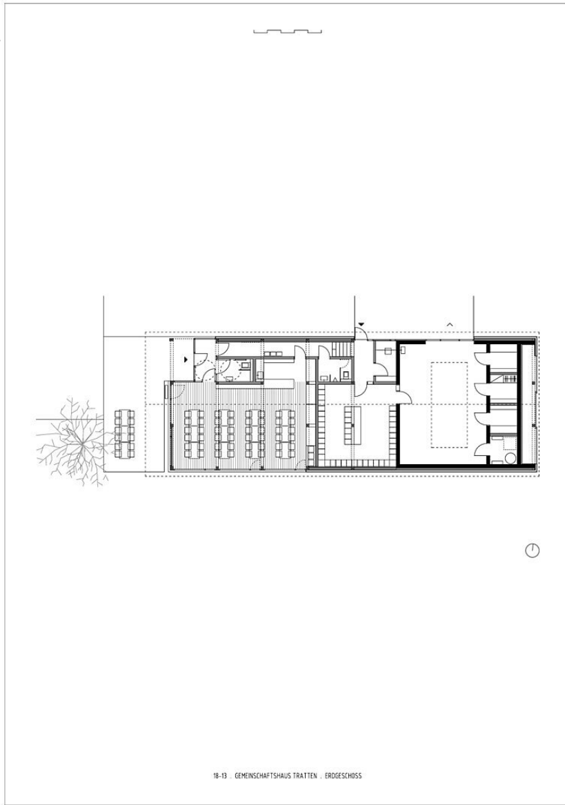
Grundriss
