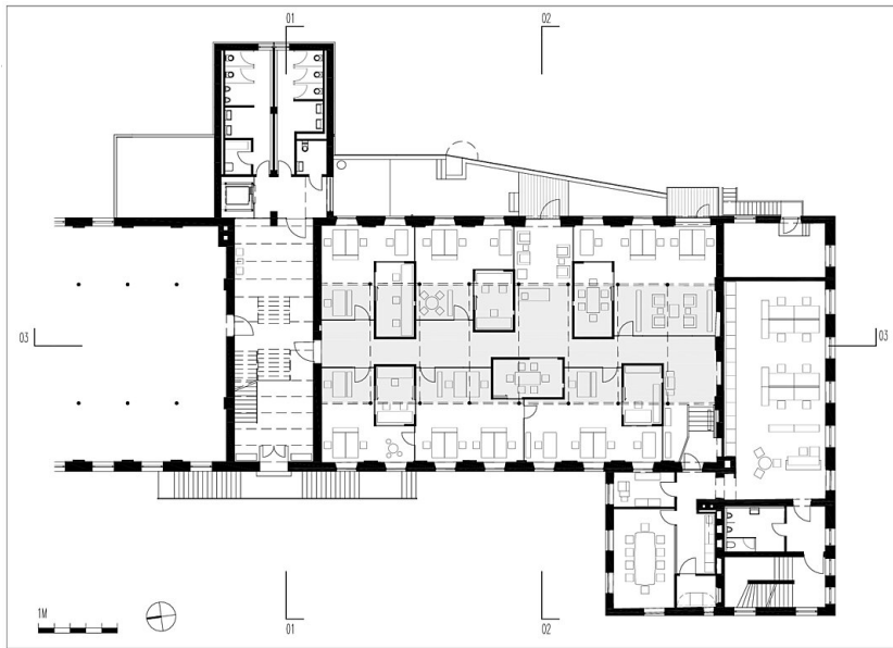
Werkstätte Walters Gebäude 6/7 - Grundriss 1. Obergeschoss
