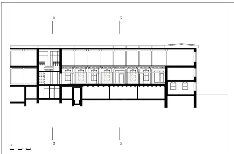
Werkstätte Wollens Gebäude 6/7 - Schnitt 03
