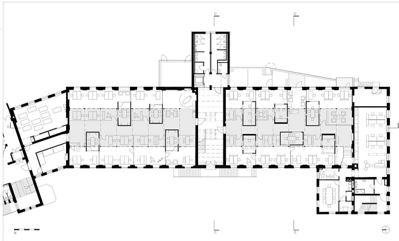
Werkstätte Walters 2. Bauabschnitt - Gebäude 5/6 Grundriss 1. Obergeschoss
