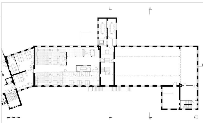
Werkstätte Walters 2. Bauabschnitt - Gebäude 5/6 Grundriss 2. Obergeschoss
