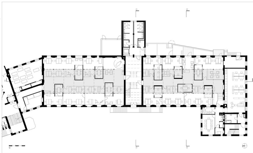
Werkstätte Walters 2. Bauabschnitt - Gebäude 5/6 Grundriss 1. Obergeschoss
