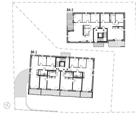
REGELGESCHOSS 1:500
