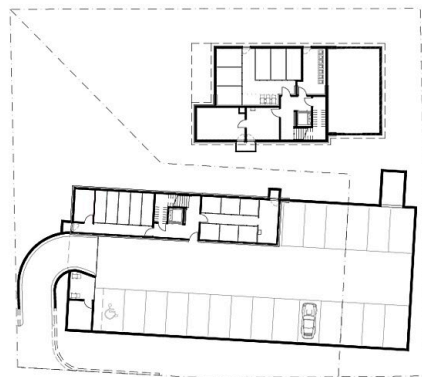
UNTERGESCHOSS 1:500
