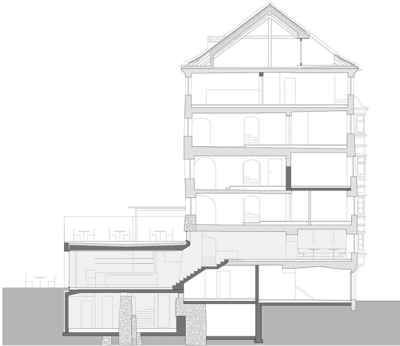
A-A 0 1 2
