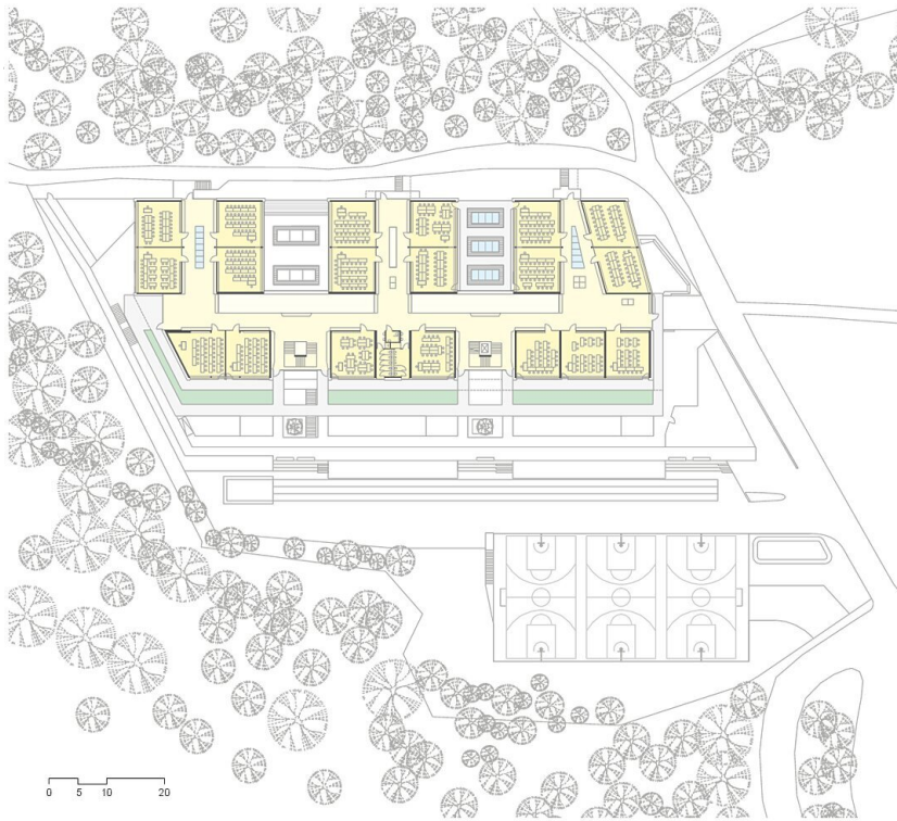
Grundriss E2
