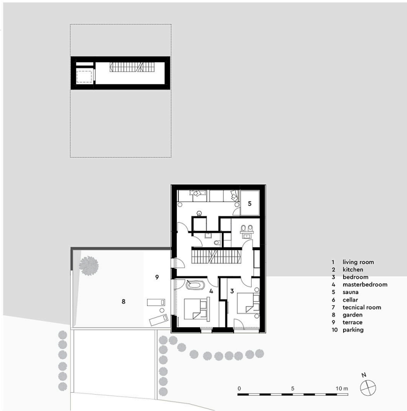
Grundriss OG1
