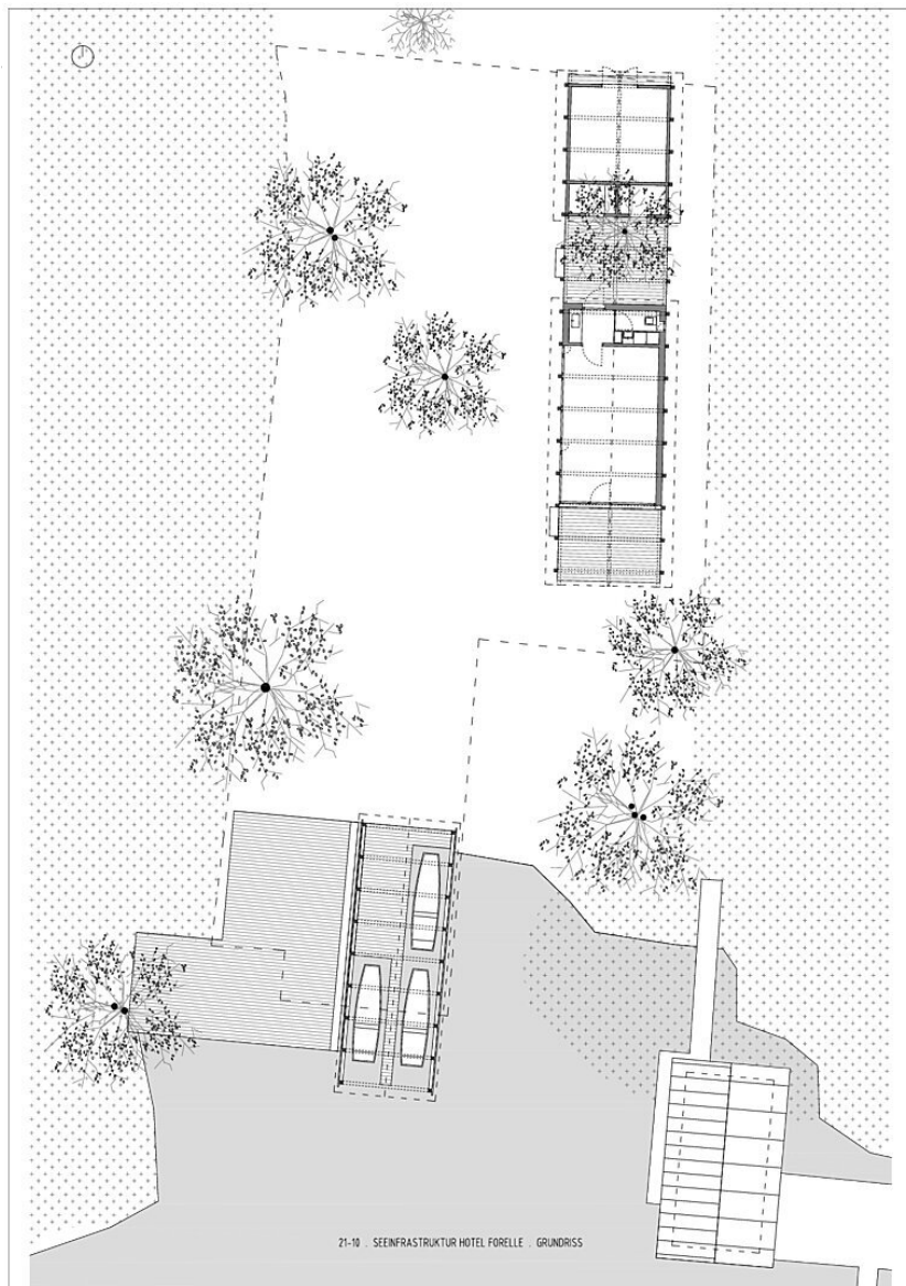
Grundriss
