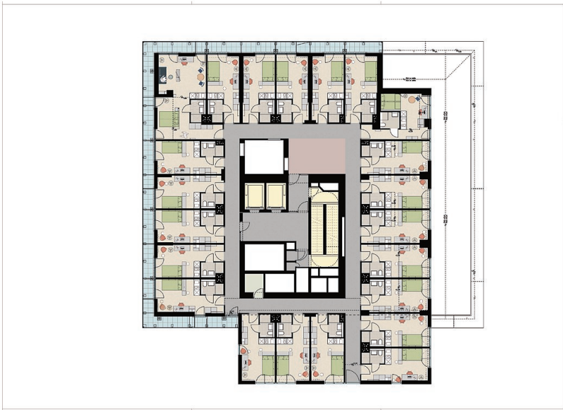
Grundriss OG21
