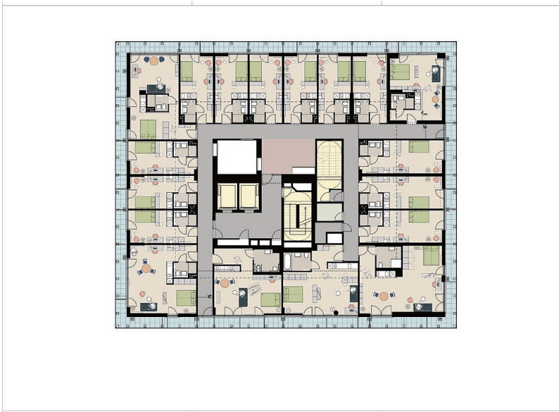
Grundriss OG34
