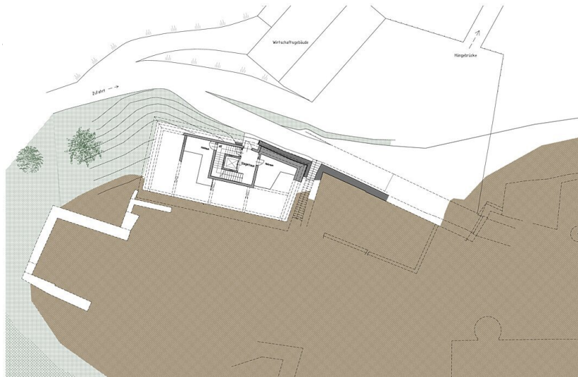
NEUBAU KULTUR- UND VERANSTALTUNGSZENTRUM BURG TRAUTSON / 6163 Mätrai am Brenner GRUNDRISS UG M. 1:200 ±0.00 = 1011.63 m.ü.A.
