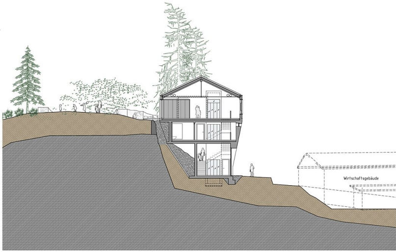
NEUBAU KULTUR- UND VERANSTALTUNGSZENTRUM BURG TRAUTSON / 6143 Matriei am Brenner SCHNITT 2-2 M. 1:200 ±0.00 = 1011.63 m.ü.A.
