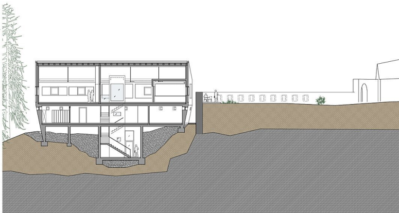
NEUBAU KULTUR- UND VERANSTALTUNGSZENTRUM BURG TRAUTSON / 6143 Matriei am Brenner SCHNITT C-C M. 1:200 ±0.00 = 1011.63 m.ü.A.
