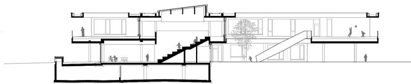
Schnitt A
