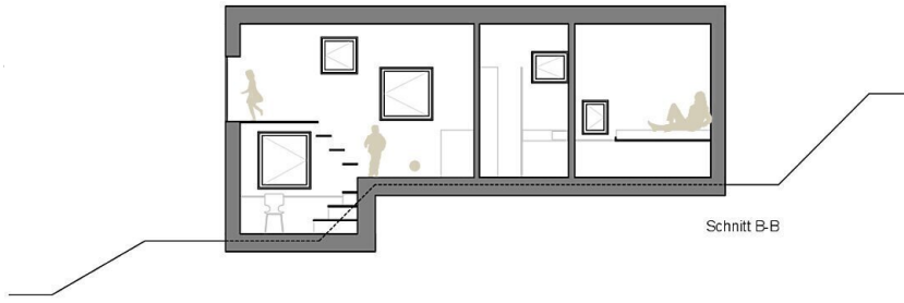
Schnitt B-B
