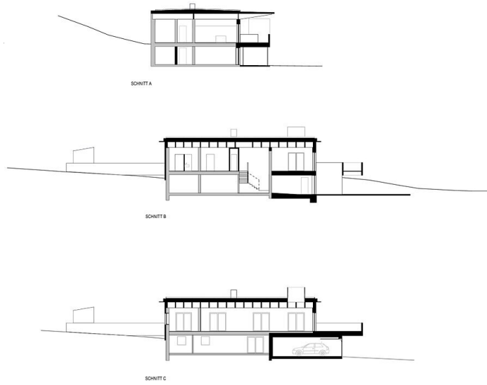
SCHNITTE [10] M 1:200 [11]
