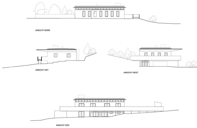
ANSICHTEN [10] M 1:200 [11]
