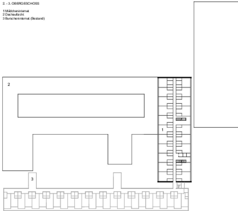
Grundriss OG3
