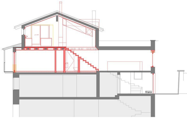
Längsschnitt Umbau
