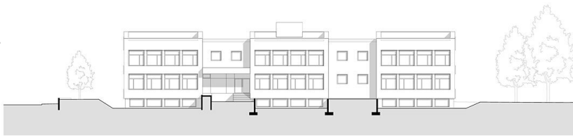
Ansicht Süden
