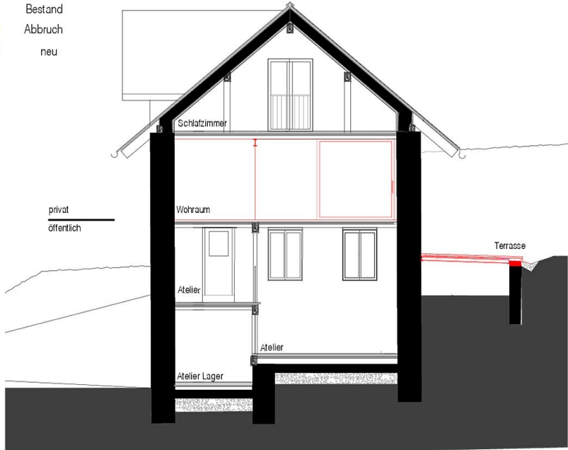
Schnitt 1 1:100
