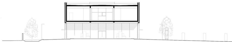
Bürogebäude mit Tankstelle GUTMANN schnitt S1 obermoser + partner zt gmbh
