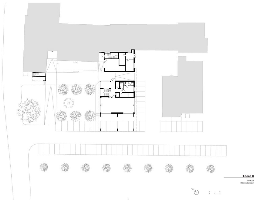
Grundriss EG
