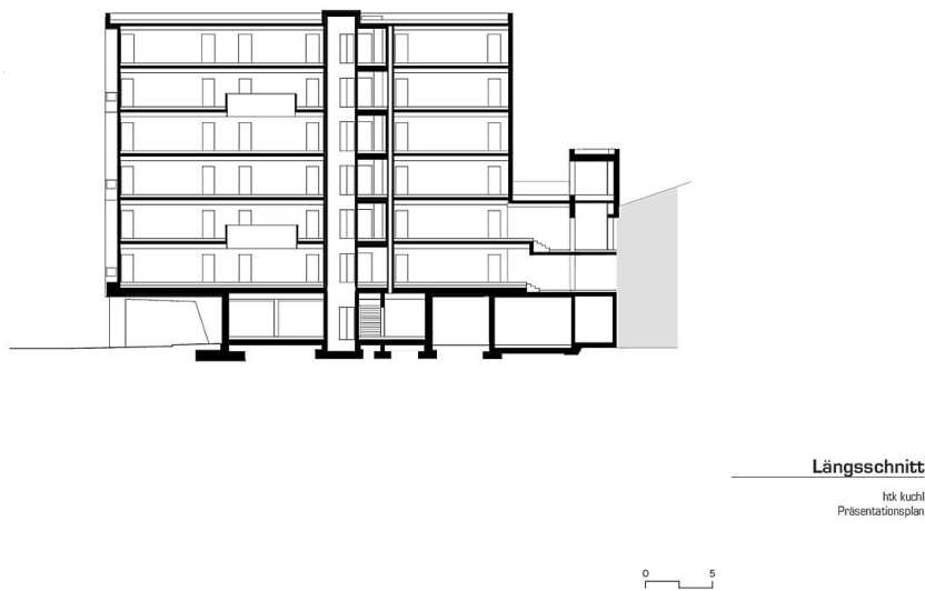
Längsschnitt
