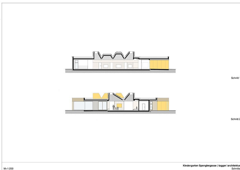
Schnitte 1, 2
