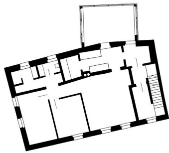
GRUNDRISS 1. OBERGESCHOSS M 1:100
