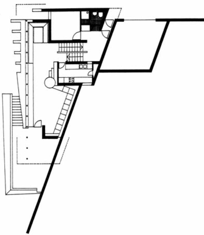
Grundriss RG
